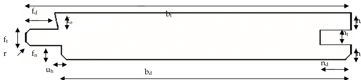
Figur 1. Dimensjoner for not og fjær.
